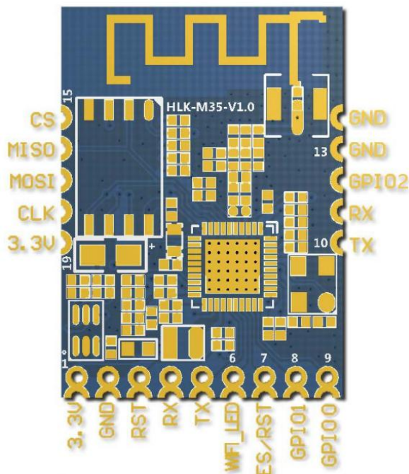
HLK-M35 管脚定义
