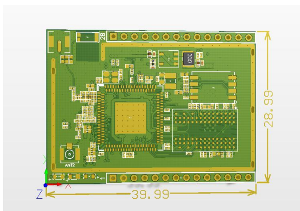
图 1 HLK-RM04N尺寸
