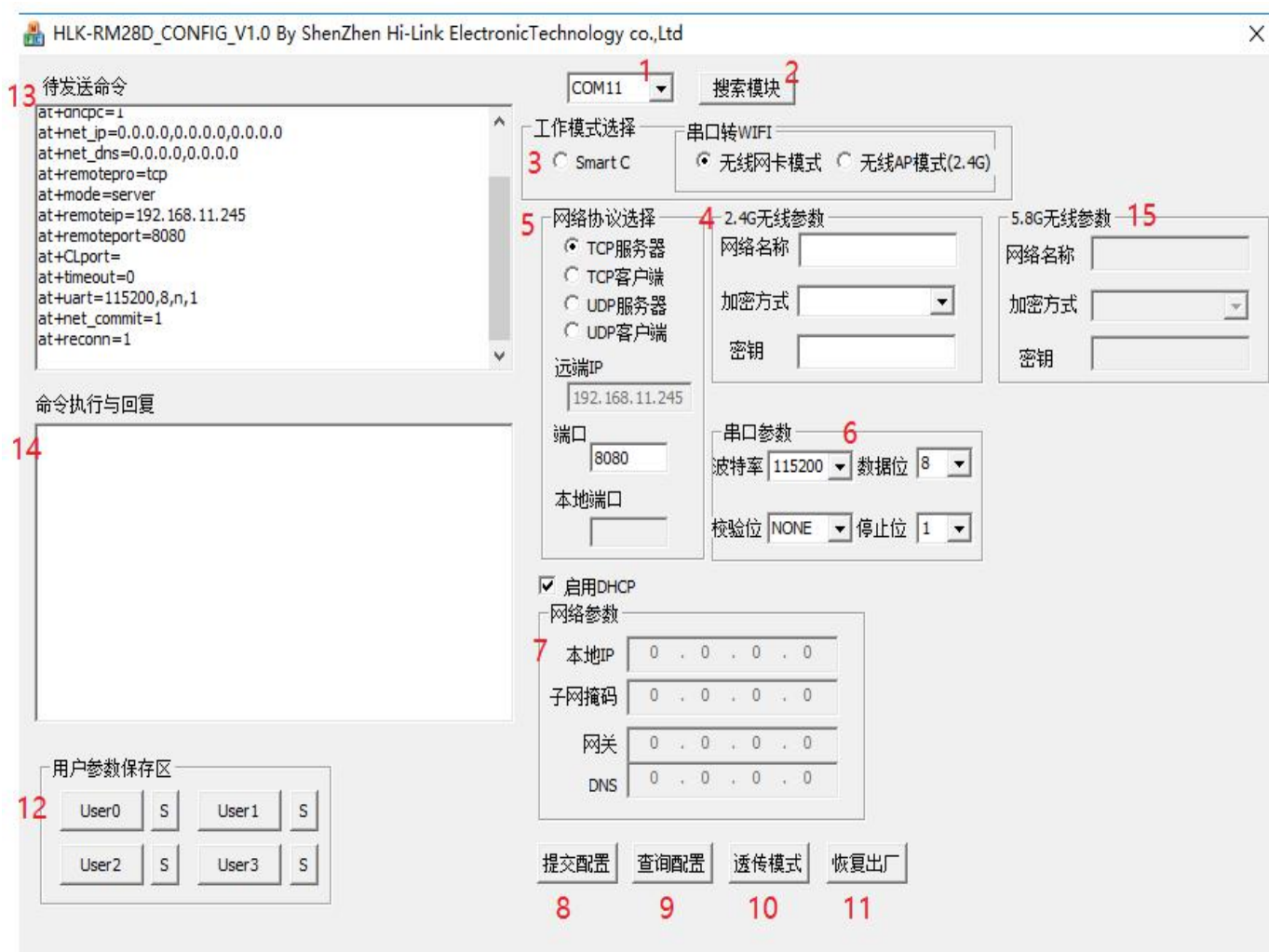
图 21. 串口配置工具界面
