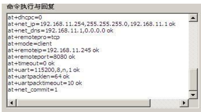
图 24. 串口配置工具指令执行
