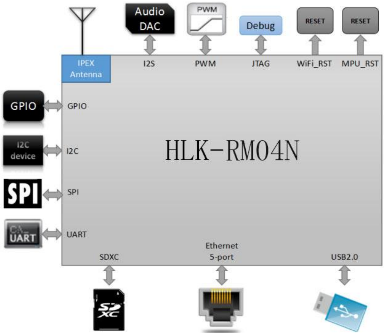
图 3 HLK-RM04N 典型外设接口图
