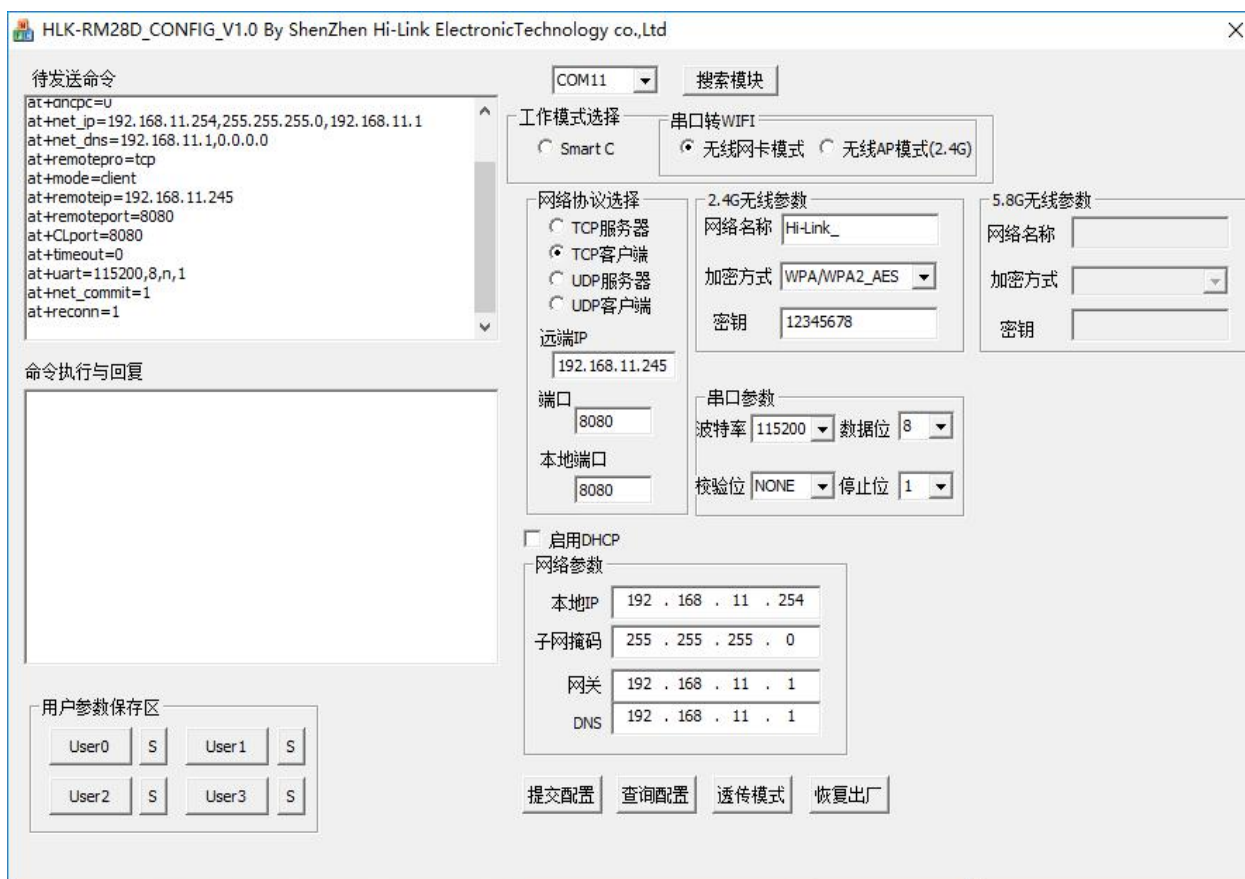
图 23. 串口配置工具生成指令
