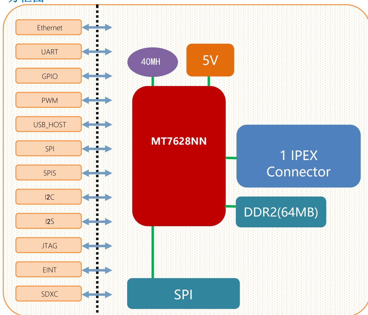
图 2 HLK-RM04N 模块架构图
