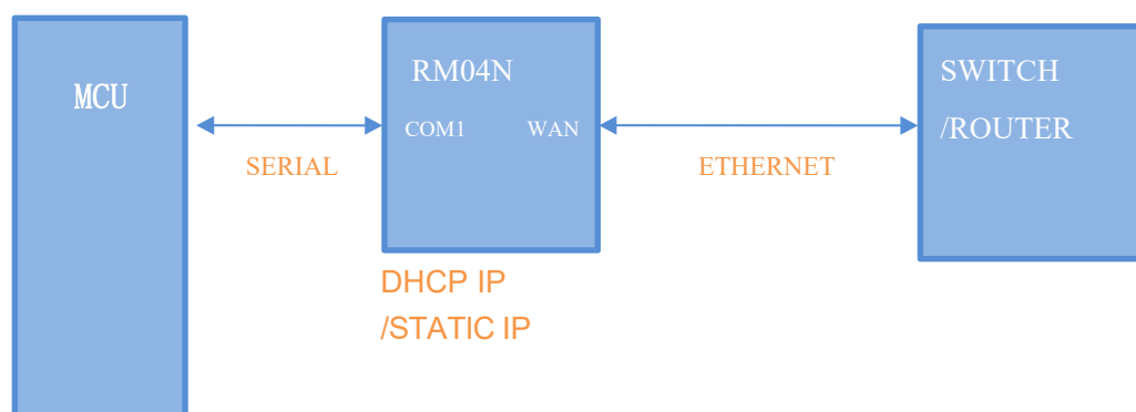
图 4. 串口转以太网
