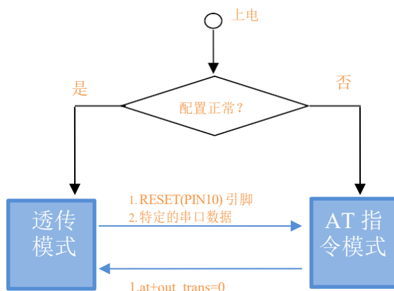
图 8 .串口工作状态转换
