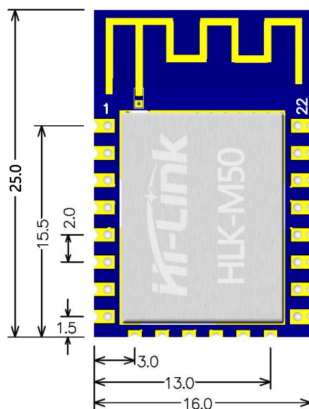
HLK-M50 尺寸图
