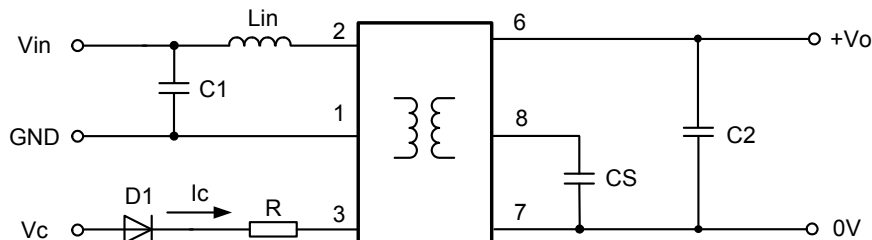
图 1 应用电路图
