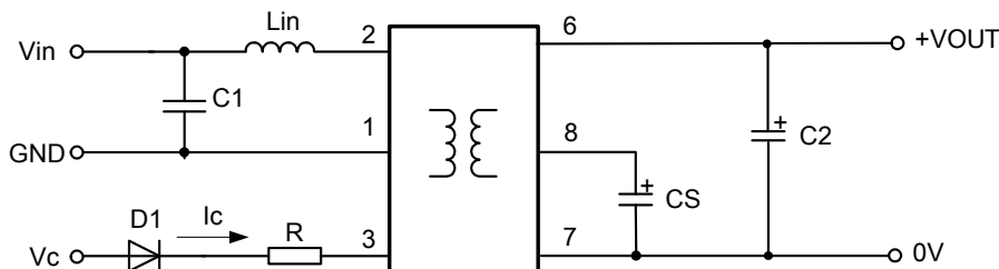
图 1 应用电路图
