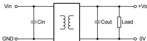
图 1 应用电路图
