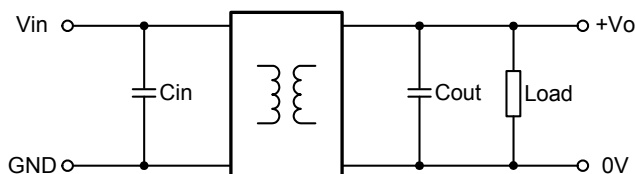
图 1 应用电路图
