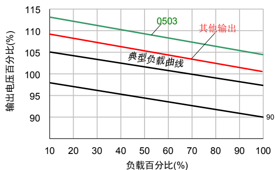
输出电压与负载关系曲线图 (标称输入电压)
