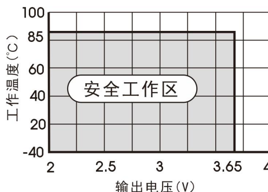
反向工作温度降额曲线
