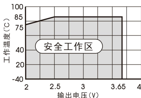
正向工作温度降额曲线
