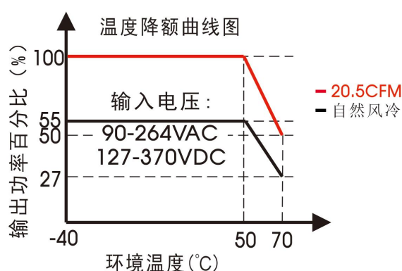
LOF350-20B15-C(满载 325W 带 20.5CFM 风扇)
