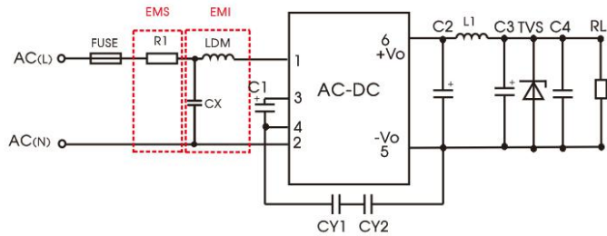
推荐电路 2
