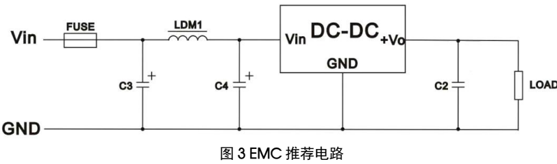
图 3 EMC 推荐电路
