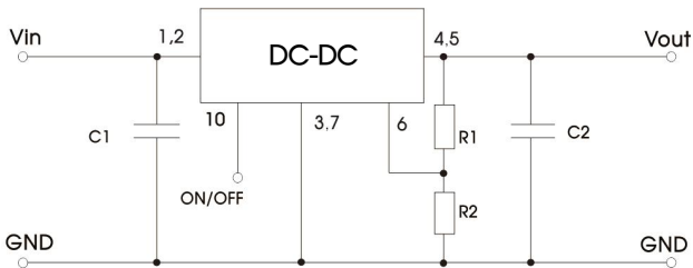
图 2 典型应用电路
