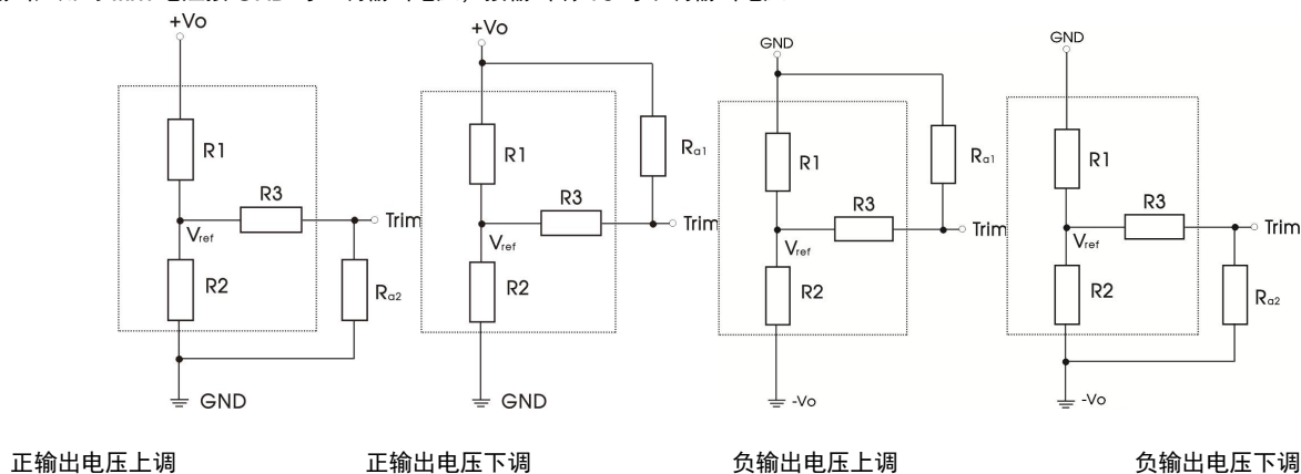
图 4 Trim 的使用电路(虚线框为产品内部)
