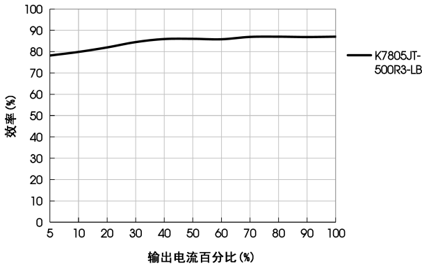
效率Vs输出负载 ( V_{in}=24\text{V} )
