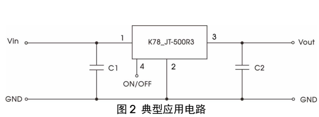
图 2 典型应用电路
