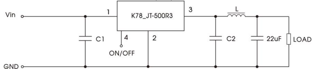
图 3 “LC”滤波应用电路
