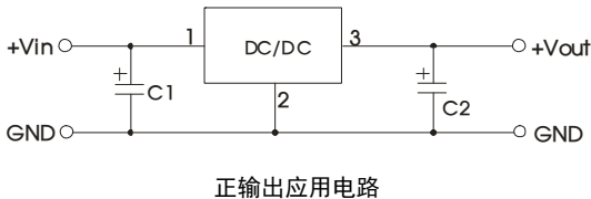
正输出应用电路
