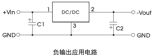
负输出应用电路
