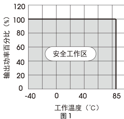
温度降额曲线图
