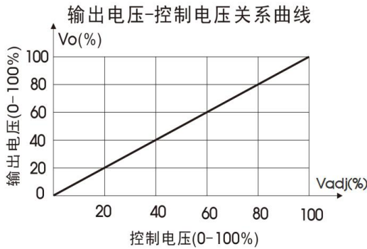
(注: 100% Vadj 等于 1.2VDC (Typ.) ) 图 4 输出电压与控制电压关系曲线
