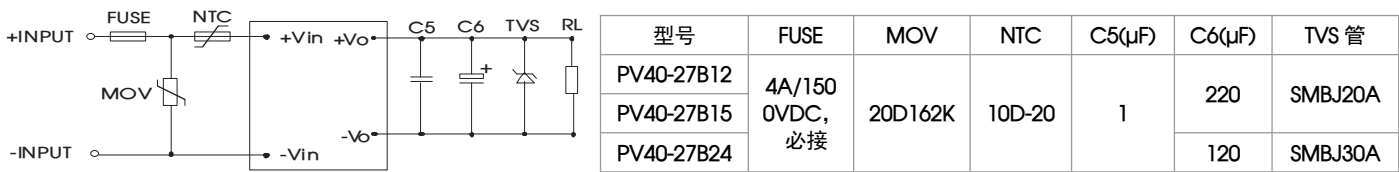
图 1: 典型应用电路
