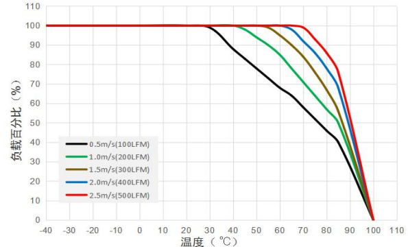
URF1D54HB-250WR3A7温度降额曲线
