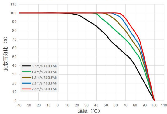
URF1D15HB-250WR3A7温度降额曲线
