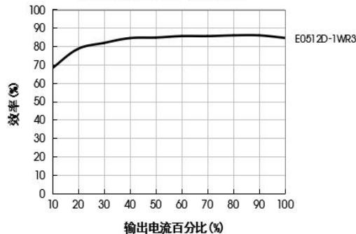
效率Vs输出负载 ( V_{in}=5\text{V} )
