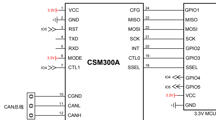
图 6 SPI 转 CAN 参考电路 (CSM300A)
