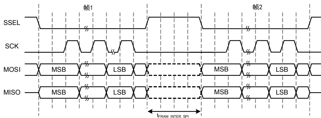
图 3 SPI 帧间隔
