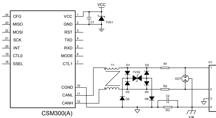
图 11 外围保护电路 2
