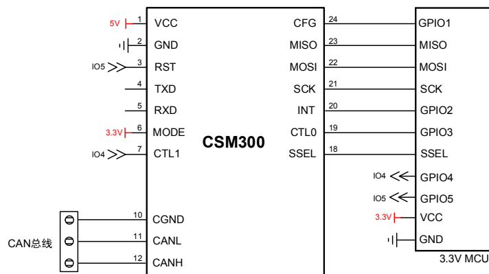
图 7 SPI 转 CAN 参考电路 (CSM300)
