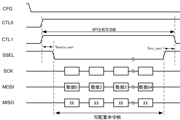
图 5 写配置
