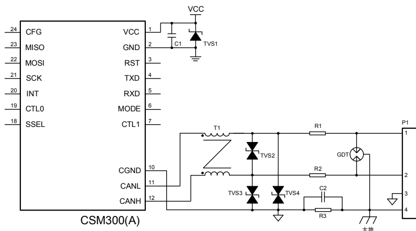
图 10 外围保护电路 1
