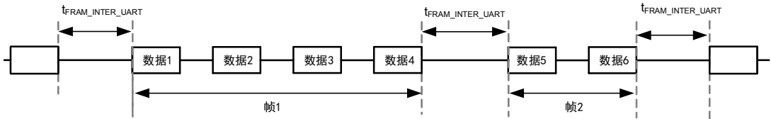
图 2 UART 帧间隔
