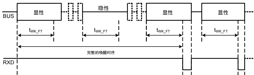
图 1 唤醒机制时序图
